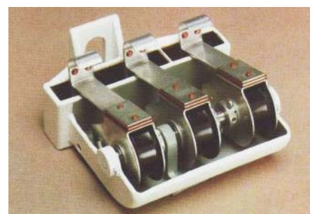
Σύστημα πίεσης: ΚC • Σχέδιο Ψηκτροθήκης. Τρεις ψηκτροθήκες τοποθετημένες παράλληλα : Γρανάζοτω κολάρο.
